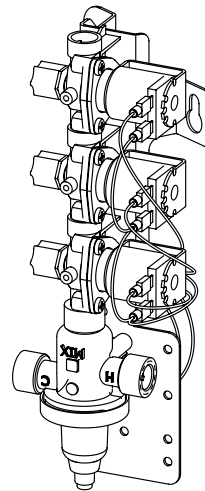
Vanne sans plomb TMA (S45-2489) représenté TL (S45-2488) est similaire Faisceau de câbles de robinet (S83-200)
